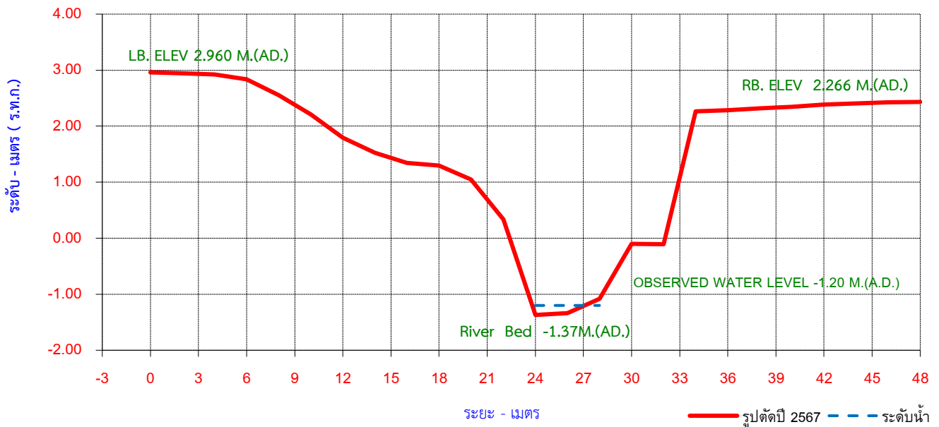
รูปตัดขวางลำน้ำ ปีนี้ 2567 สถานี Sw.16 ห้วยแม่สอด อ.แม่สอด จ.ตาก
